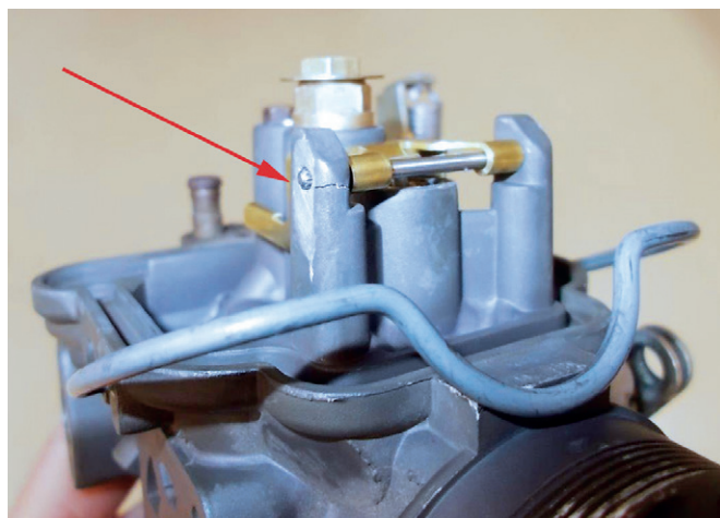
Auf der Seite, wo der Stahlstift (Splint) seine Zahnungen hat, um diesen am Verrutschen zu hindern, war ein markanter Riss im Gussgehäuse erkennbar
